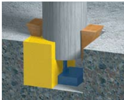
Стаканы сборных колонн
